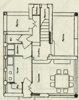
PLANTA BAJA Escala 1/50
