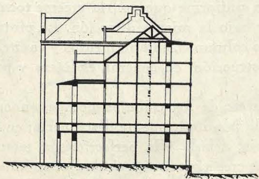
SANATORIO EN FUENFRÍA (GUADARRAMA). — SECCIONES.
