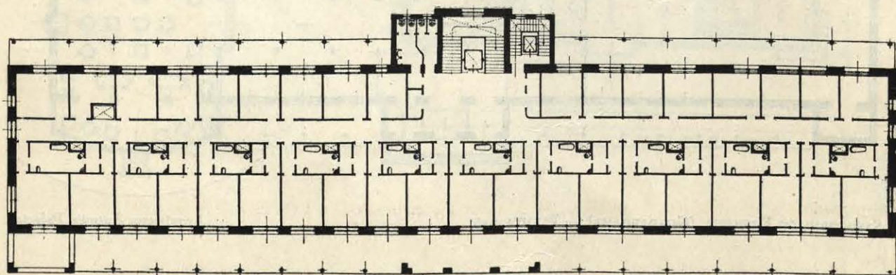
SANATORIO EN FUENFRÍA (GUADARRAMA). — PLANTAS 1 Y 2.
