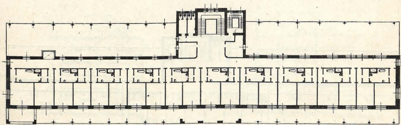
SANATORIO EN FUENFRÍA (GUADARRAMA). — PLANTA 3.
