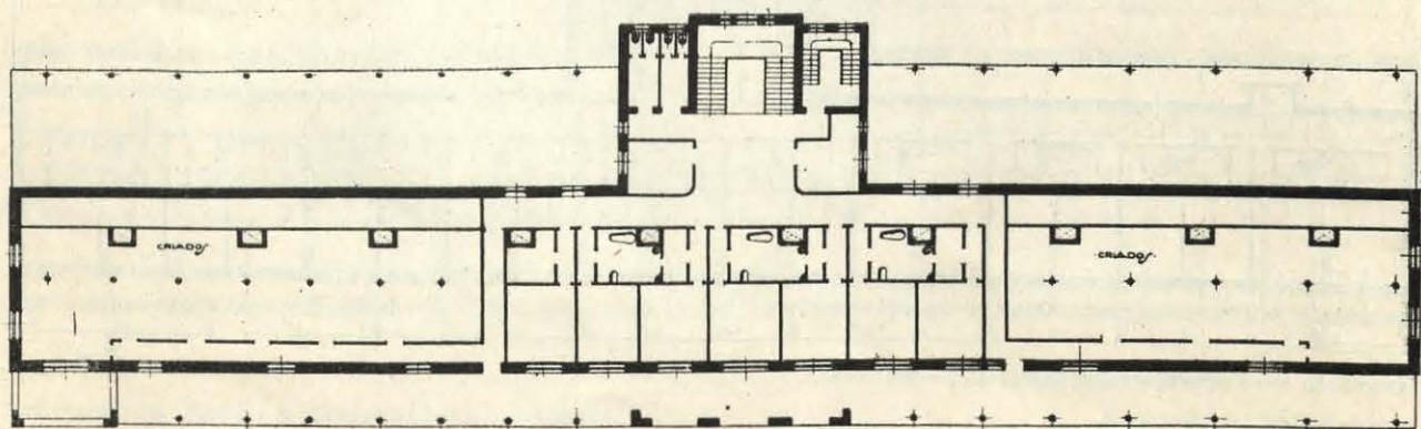
SANATORIO EN FUENFRÍA (GUADARRAMA). — PLANTA 4.
