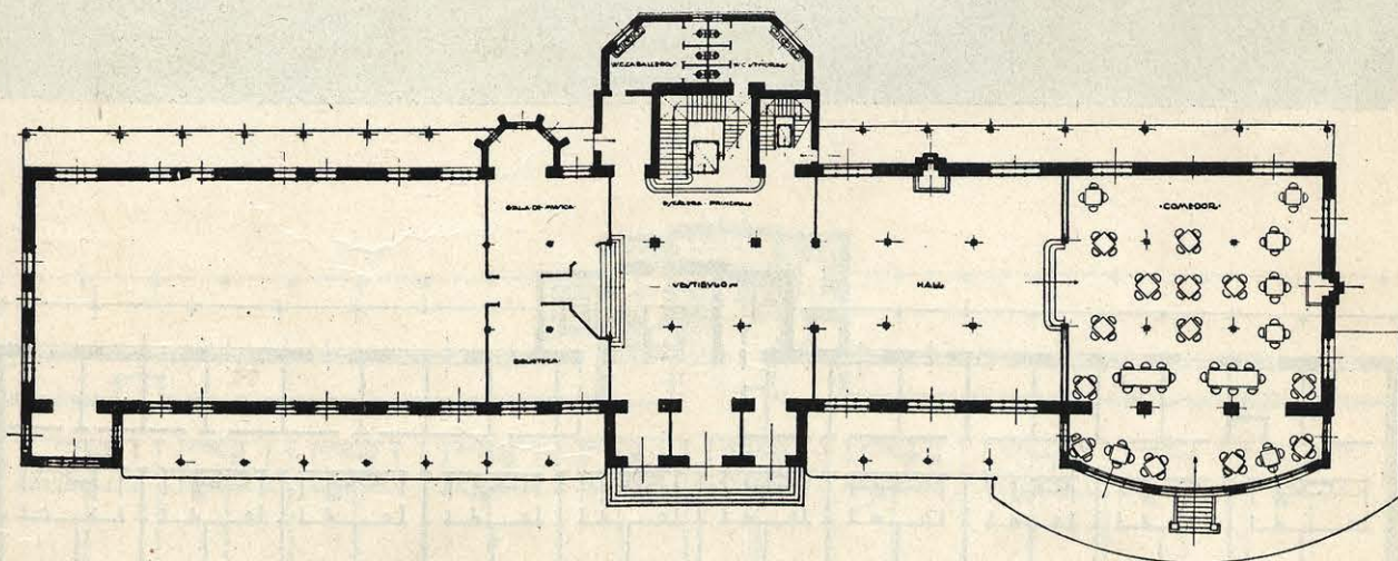
SANATORIO EN FUENFRÍA (GUADARRAMA). — PLANTA BAJA.
